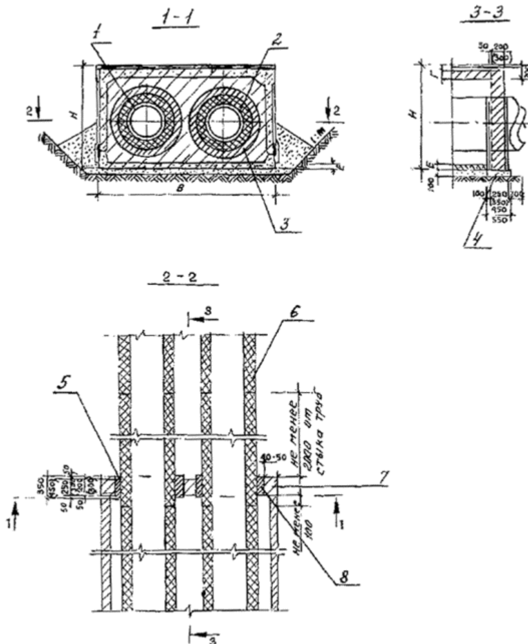
Рис. 4. Конструкция сопряжения бесканальной прокладки с канальной:
