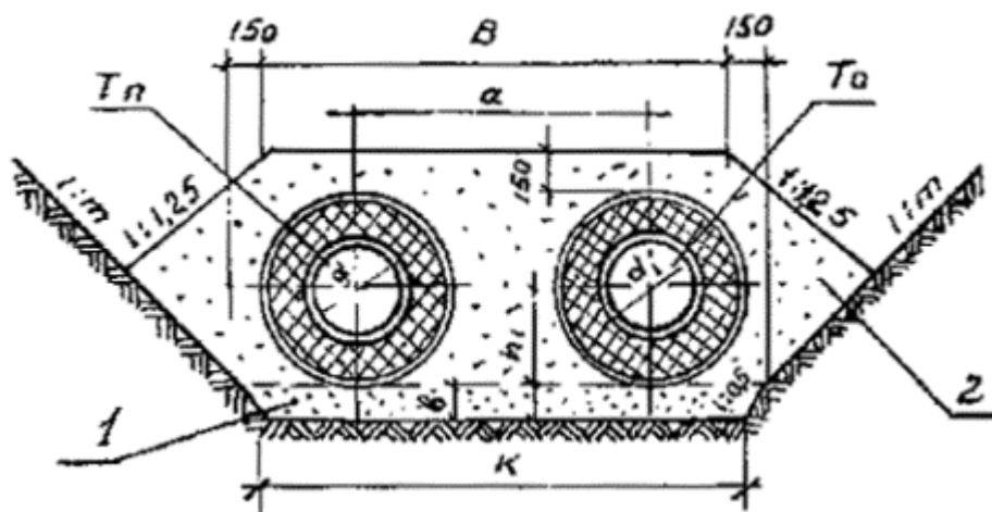
Рис. 2. Сечение двухтрубной бесканальной прокладки:
