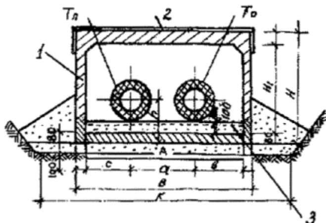
Рис. 3. Сечение двухтрубной прокладки в монолитном канале:
