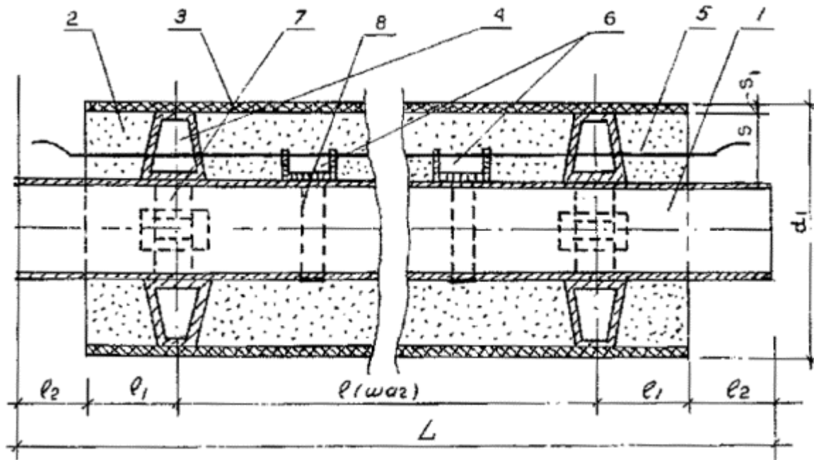
Рис. 1. Индустриальная конструкция теплоизоляции труб:
