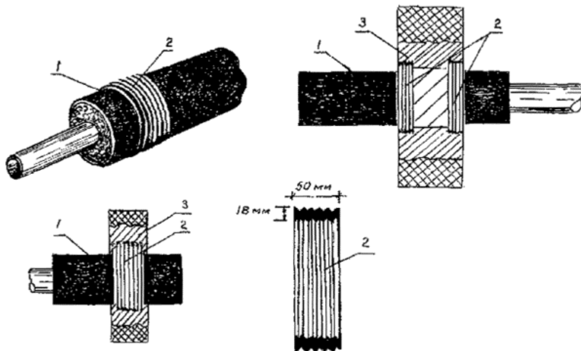
Рис. 6. Конструкция прохода теплопроводов сквозь стены фундамента зданий:
