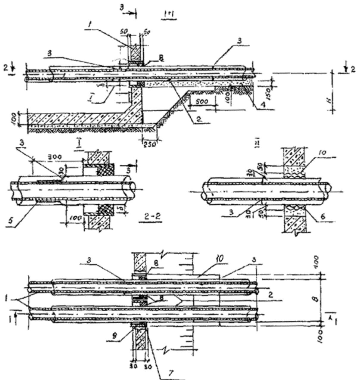
Рис. 5. Конструкция прохода теплопроводов через стены камер, камер-павильонов:
