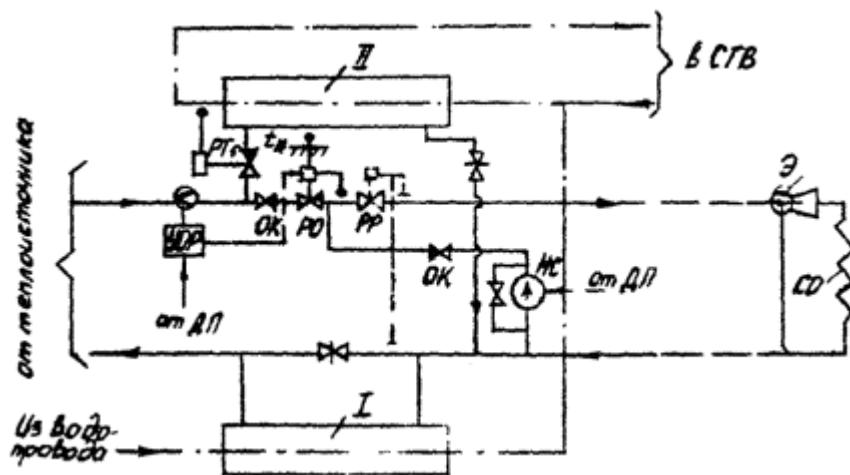
Рис. 1. Технологическая схема ЦТП со смешанной схемой присоединения водонагревателя горячего водоснабжения, автоматическим регулированием отпуска теплоты и зависимым присоединением систем отопления:
