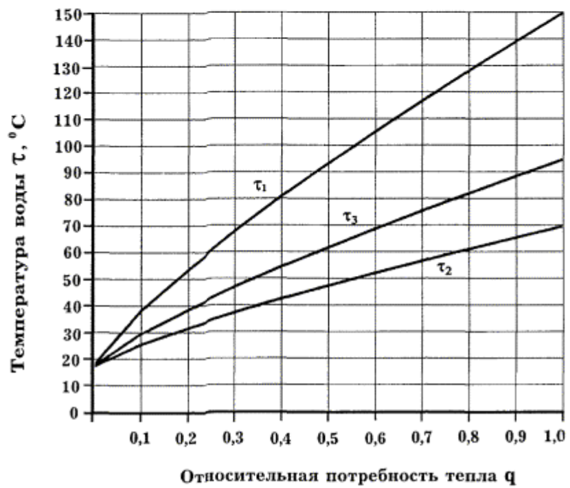
Рис. 3. Скорректированный график № 1 регулирования отпуска тепловой энергии
